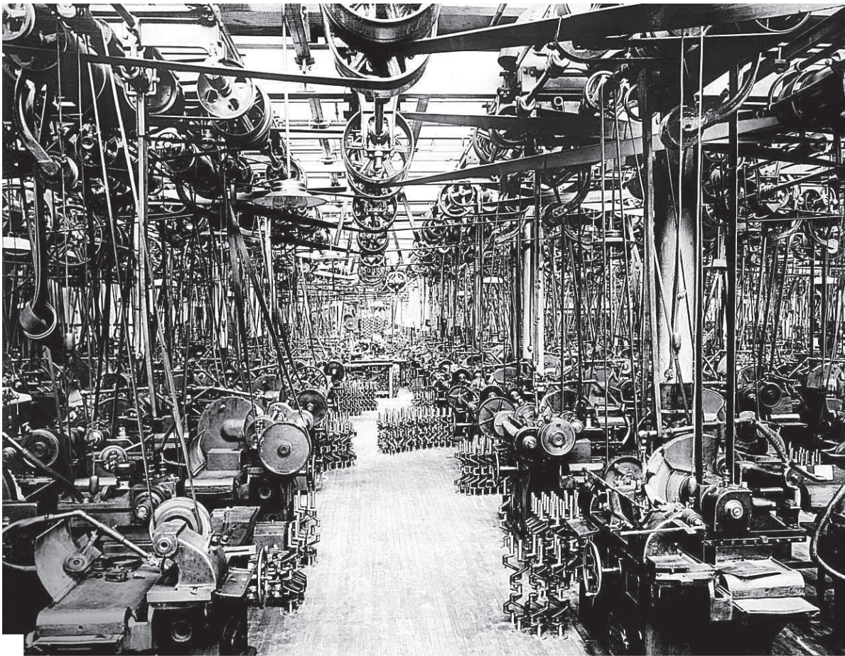
■ Станки в шлифовальном отделе
