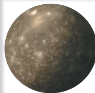
Каллисто
