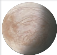
Европа
