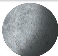
Рея
