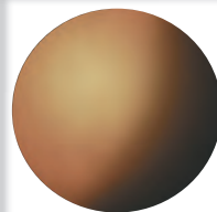
Титан
