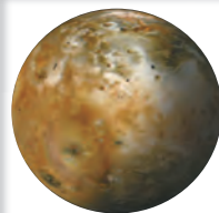
Ио
