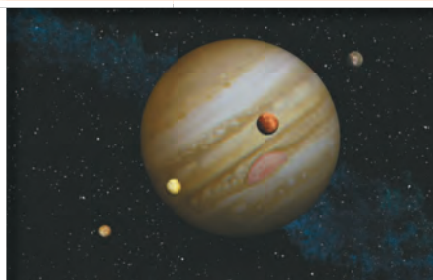
Юпитер
