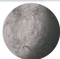
Титания
