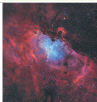
Туманность Орел
