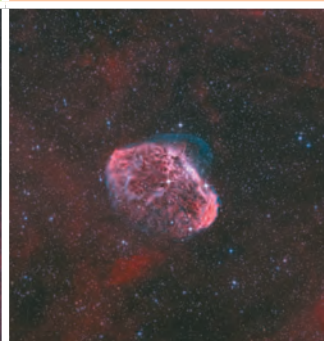
Туманность Полумесяц
