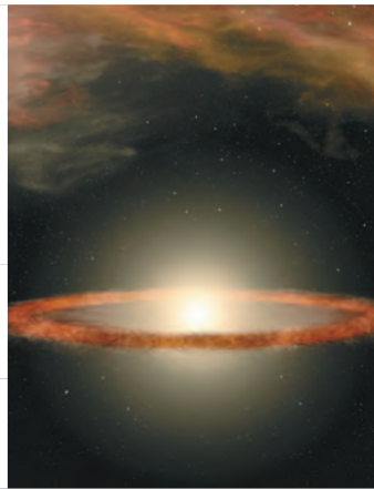
Взрыв сверхновой звезды
