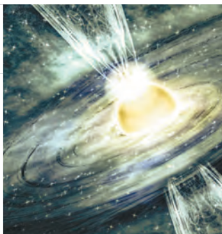
Модель разделения материи и энергии
