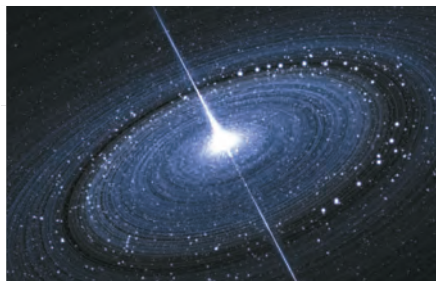
Звездный диск вокруг сверхмассивной черной дыры
