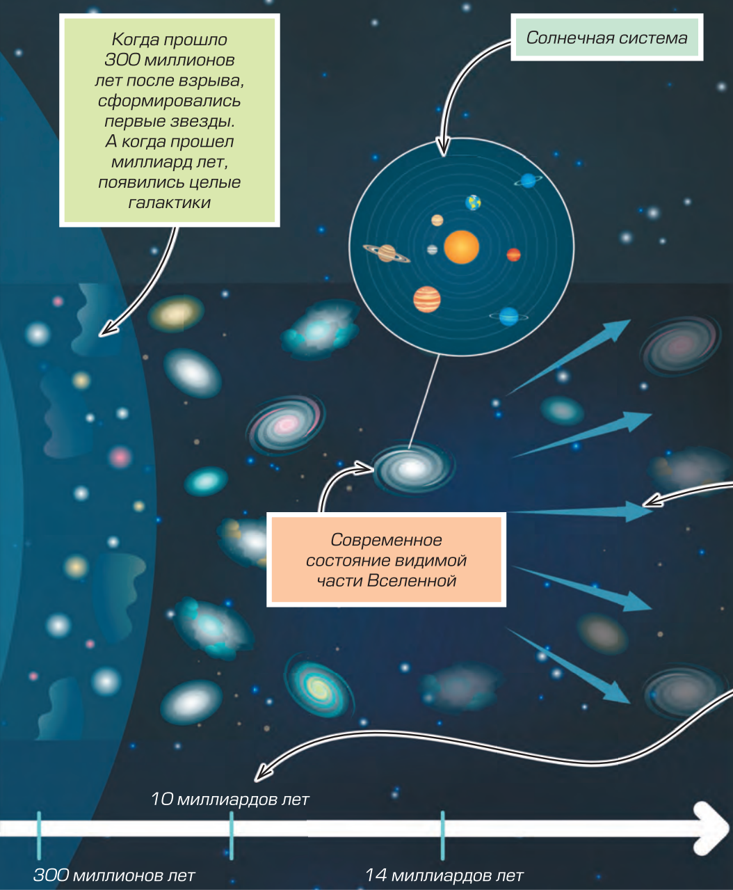
Глубокий космос
