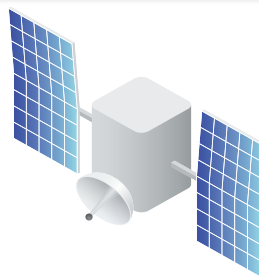
Спутник
