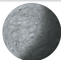
Япет
