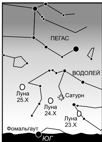
Рис. 7. Луна и Сатурн вечером 23–25 октября
