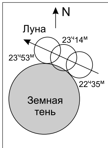
Рис. 8. 28 октября — частное лунное затмение
