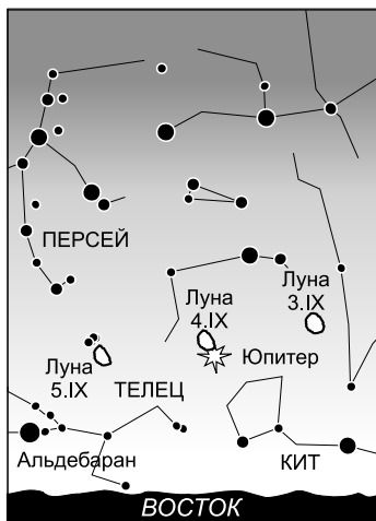
Рис. 3. Луна и Юпитер вечером 3–5 сентября
