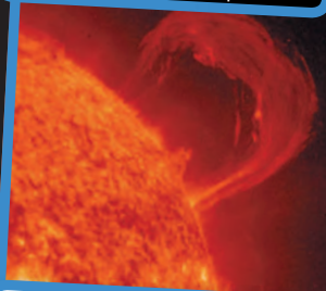
ПРОТУБЕРАНЦЫ
