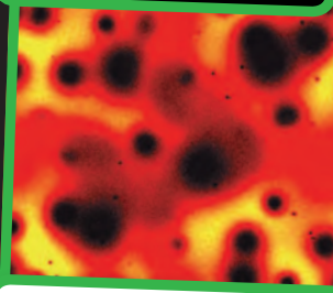
СОЛНЕЧНЫЕ ПЯТНА
