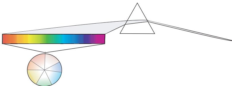
Призма Ньютона
