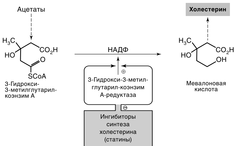
Рис. 1.5. Локализация действия ингибиторов 3-гидрокси-3-метилглутарилкоэнзим А-редуктазы. НАДФ — никотинамидадениндинуклеотидфосфат
