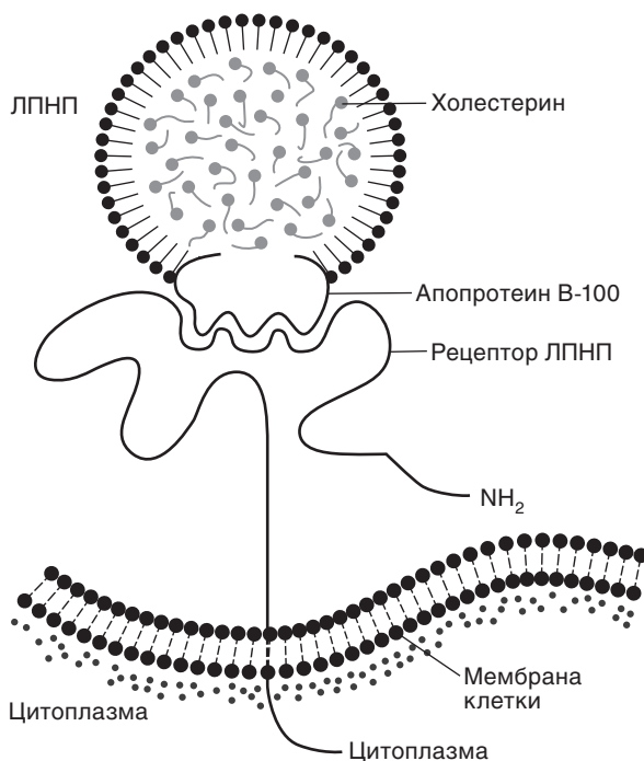
Рис. 1.4. Схематическое представление комплекса, состоящего из рецептора липопротеина низкой плотности на мембране клетки и липопротеина низкой плотности липопротеида. NH 2 — одновалентная группа
