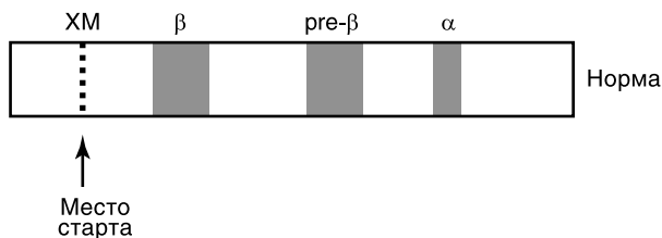
Рис. 1.1. Электрофоретический профиль липопротеинов (схема)
