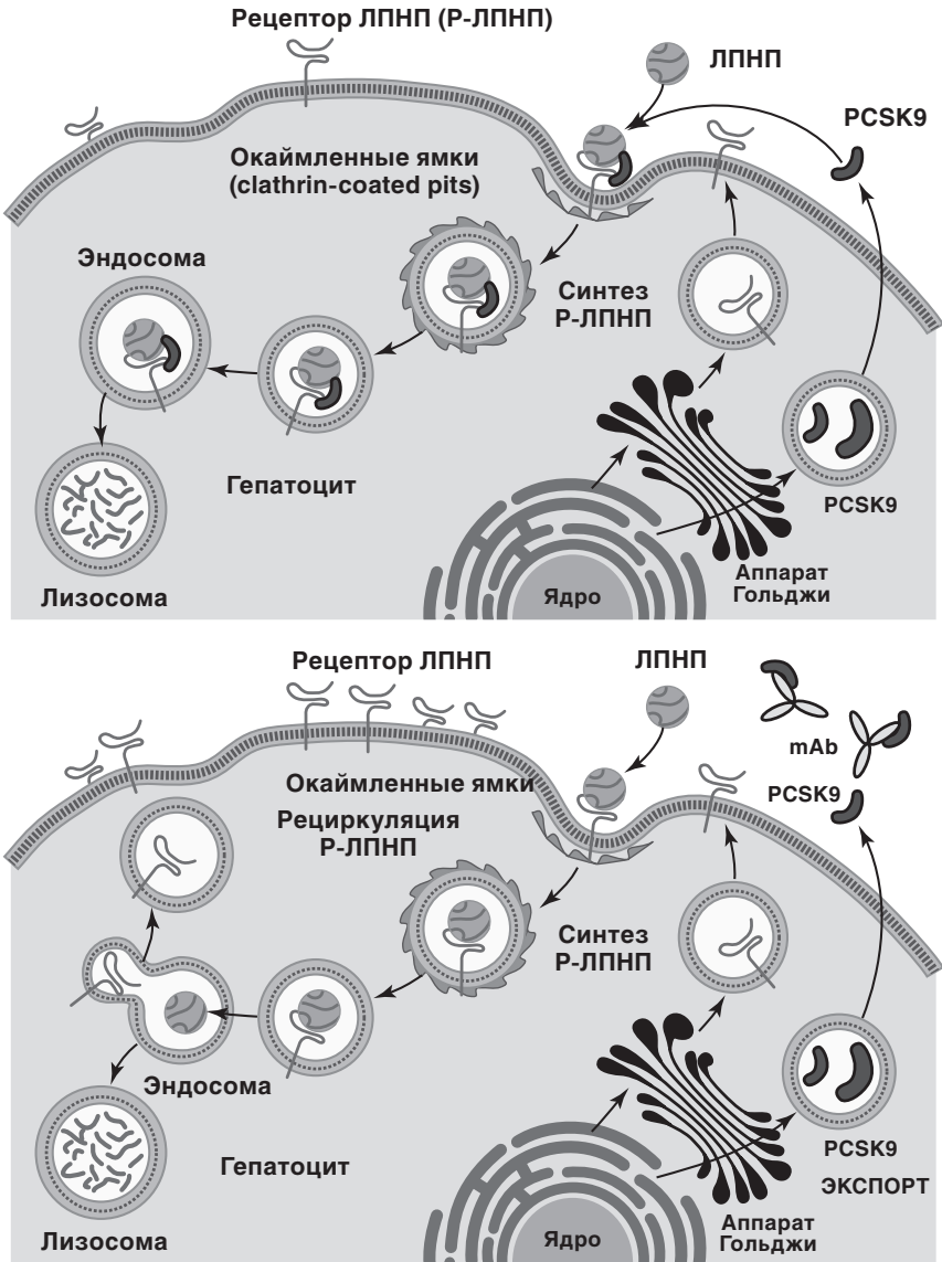
Рис. 1.7. Участие пропротеин конвертаза субтилизин/кексин в регуляции активности рецепторов липопротеинов низкой плотности [269]. mAb — моноклональные антитела к PCSK9
