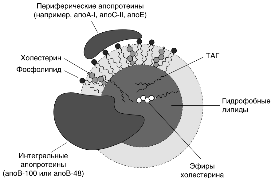
Рис. 1.3. Схематическое изображение структуры липопротеиновой частицы. ТАГ — триацилглицеролы, нейтральные жиры
