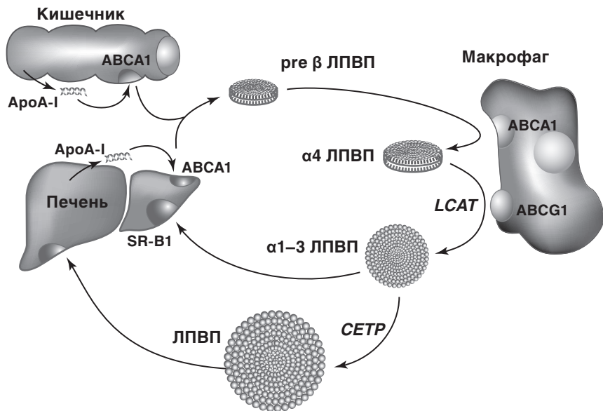
Рис. 1.8. Обратный транспорт холестерина из периферических тканей в печень. ABCA1 — АТФ-связывающий кассетный транспортер; ABCG1 — член 1 подсемейства G АТФ-связывающей кассеты; ЛПВП — липопротеины высокой плотности; LCAT — лецитин-холин ацилтрансфераза; CETP — белок, переносящий эфиры холестерина
