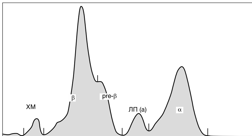
Рис. 1.2. График денситометрии липопротеидов в полиакриламидном геле. ЛП (а) — липопротеид а
