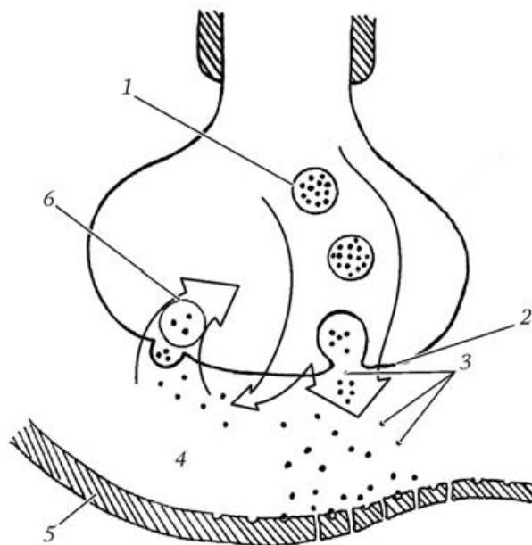
Рис. 8. Ультраструктура синапса:
