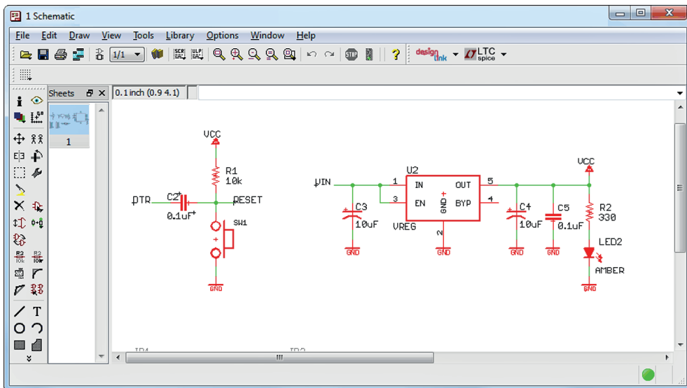
Рис. 1.1. Редактор схем EAGLE
