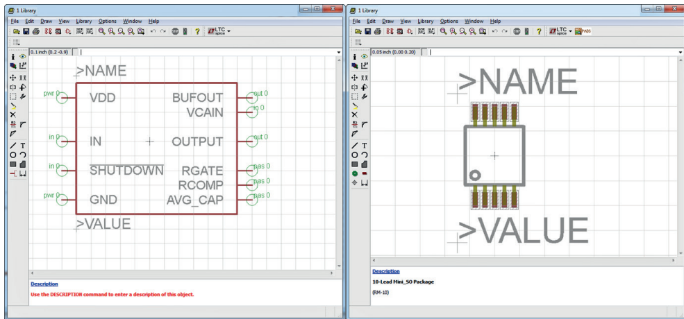
Рис. 1.3. Редакторы компонентов EAGLE
