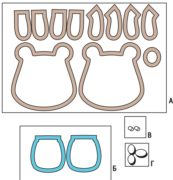
План раскладки лекал на ткани
