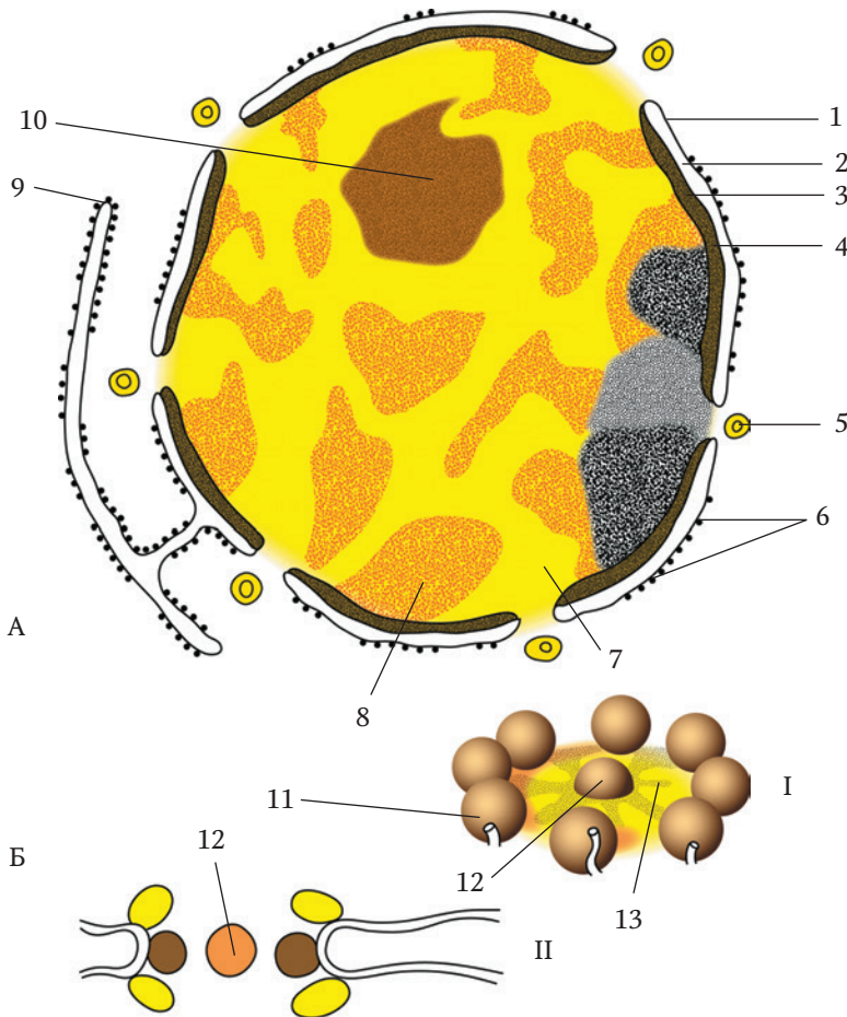
Рис. 8. Ядро клетки: А — ядро: 1 — наружная мембрана кариотеки (наружная ядерная мембрана); 2 — перинуклярное пространство; 3 — внутренняя мембрана кариотеки (внутренняя ядерная мембрана); 4 — ядерная пластинка; 5 — поровый комплекс; 6 — рибосомы; 7 — нуклеоплазма (ядерный сок); 8 — хроматин; 9 — цистерна зернистой эндоплазматической сети; 10 — ядрышко; Б — поровый комплекс: I — пространственная реконструкция; II — схема основных структур; 11 — периферическая гранула; 12 — центральная гранула; 13 — диафрагма поры
