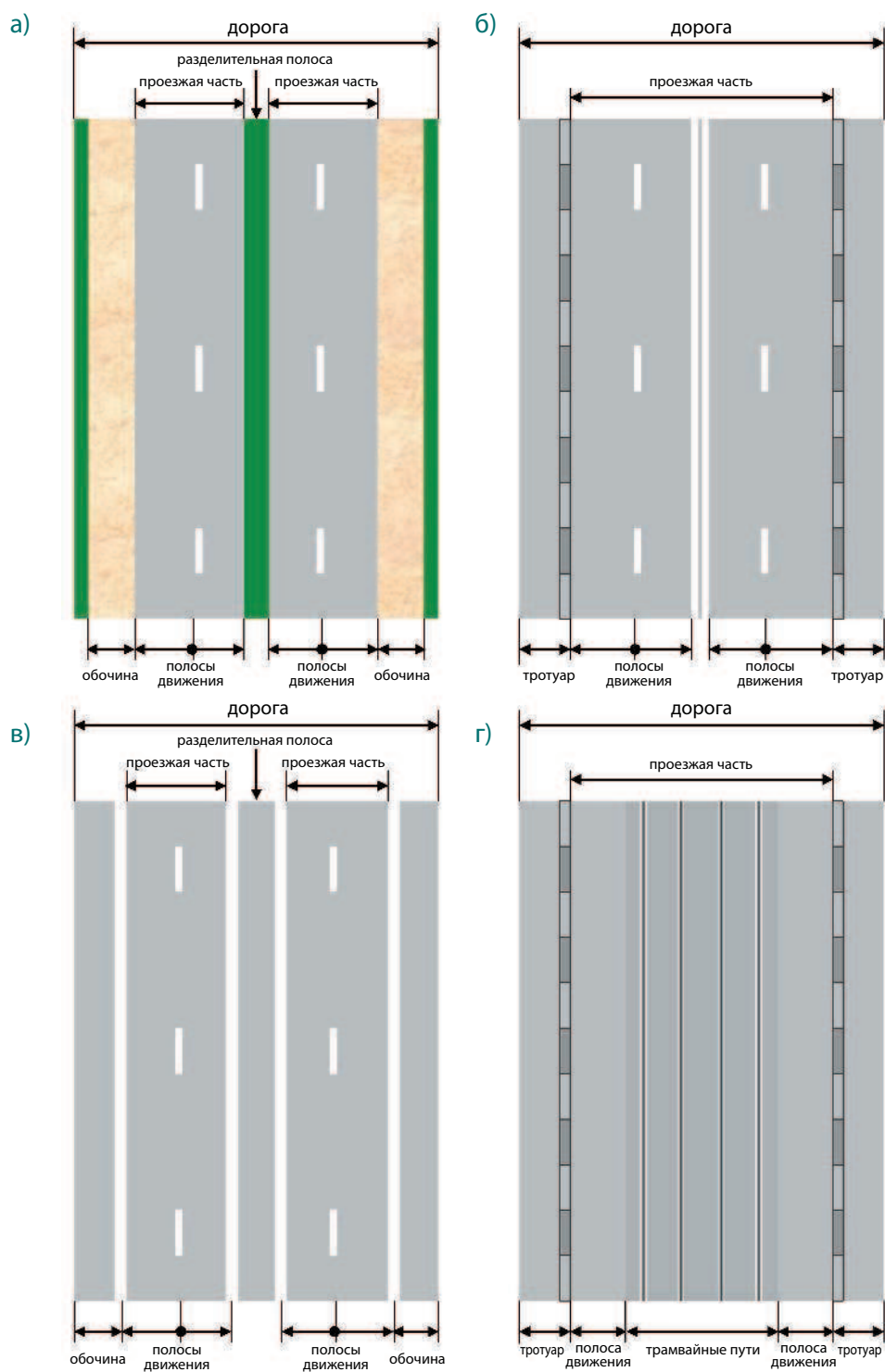
РИС. 1 Элементы дороги (1.2)
