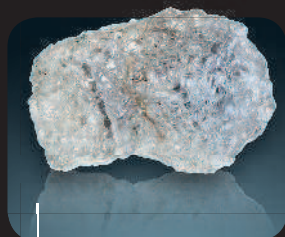
Природный кристалл алмаза низкого качества (Африка)
