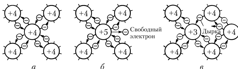
Рис. 1.2. Кристаллическая структура чистого полупроводника ( а ), полупроводника с донорной ( б ) и акцепторной ( в ) примесью
