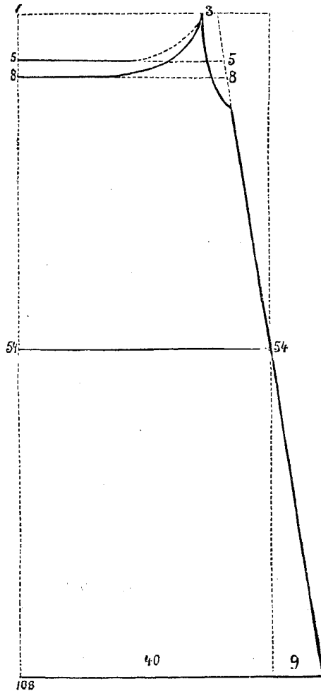
Черт. 7. Станъ рубашки съ круглою кокеткою.
