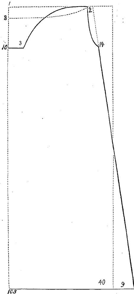
Черт. 16. Рубашки съ кокеткой спереди съ застежкой.
