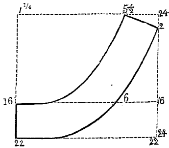
8-й черт. круглой кокетки.
