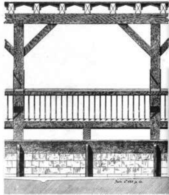
Детали устройства нормовыхъ ящиковъ.
