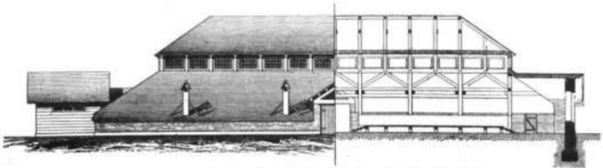
Продольный разръзъ.
