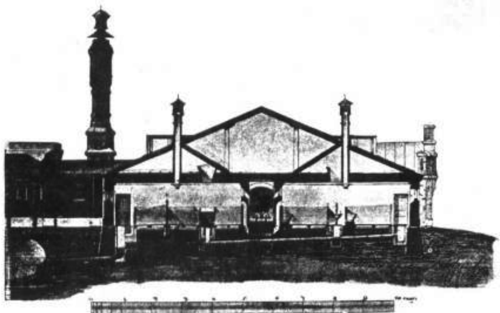
Разрѣзъ кровли.
