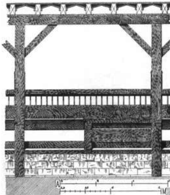
Главный фасадъ.
