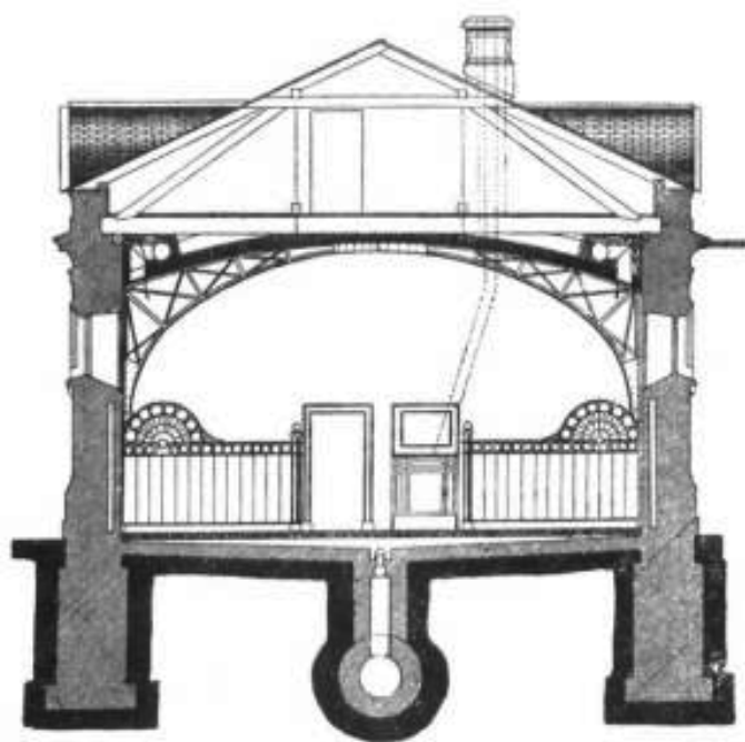
Поперечный разрезъ.
