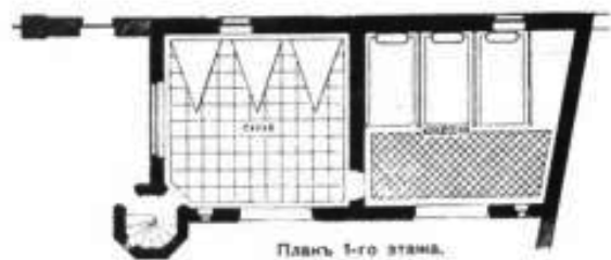
Планъ 1-го этажа.
