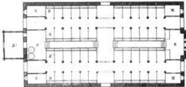
Детальный планъ.
