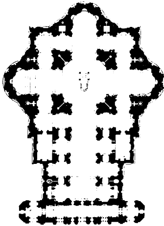
ПЛАНЫ СОВОРА СВ. ПЕТРА ВЪ РИМѢ.
