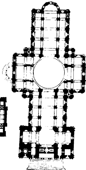
ПЛАНЪ СБОРА СП. ПАВЛА ВЪ ЛОНДОНЪ
