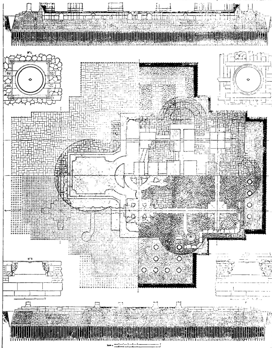
ПЛАНЫ СКАМ ПОДЪ ФУНДАМЕНТОМЪ СОВОРА
