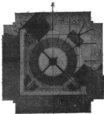
Планъ железныхъ стропилъ для поддержки большого колокола
