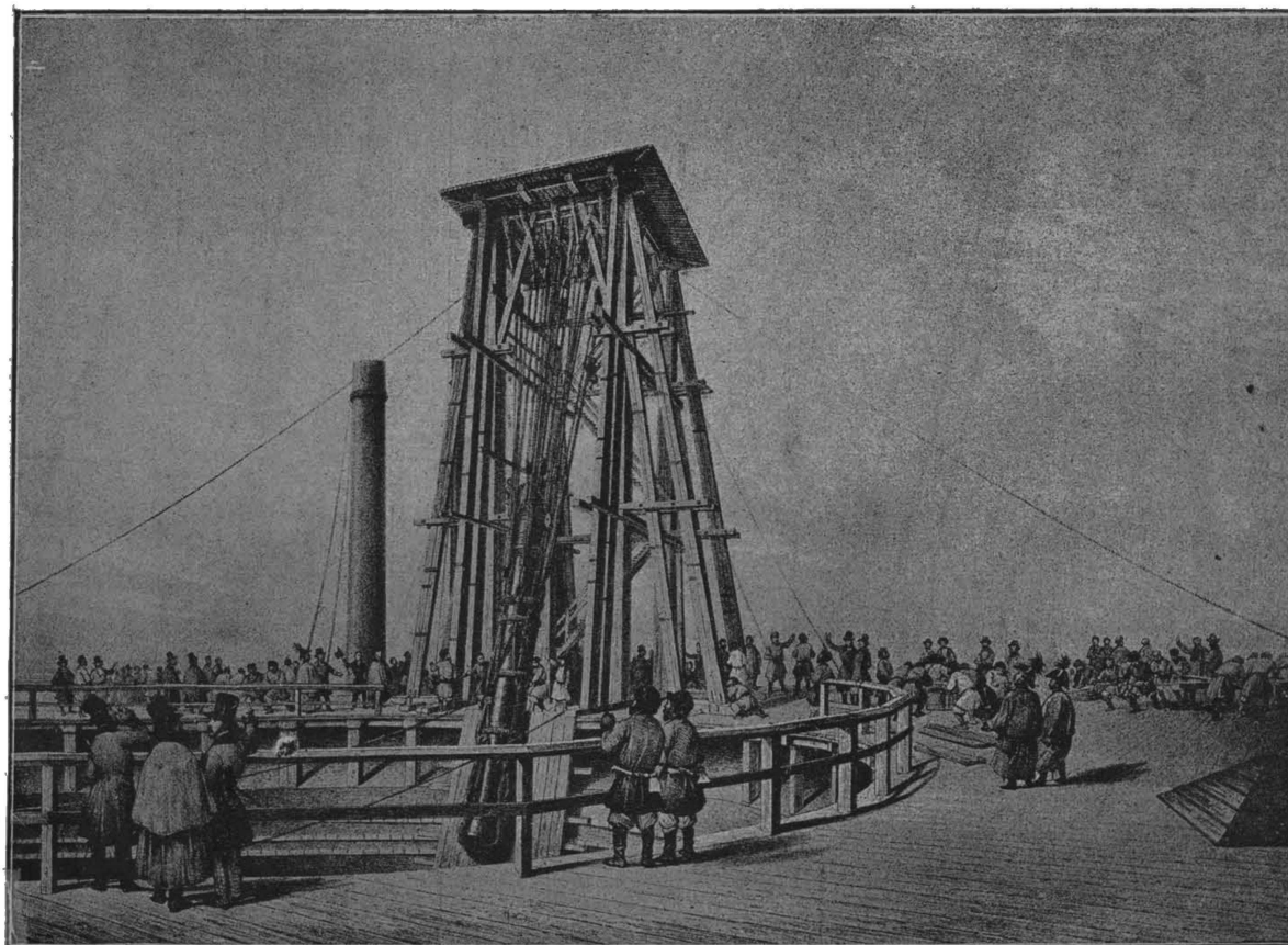
УСТАНОВКА КОЛОНЫ НА АКСИУ
