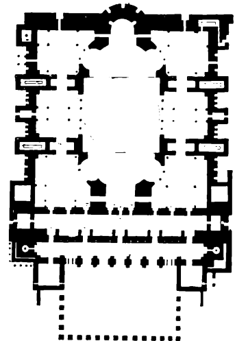
ПЛАТЪ МЕЧЕТИ АЛЯ-СОФИЯ ВЪ КОНСТАНТИНОПОЛѢ.
