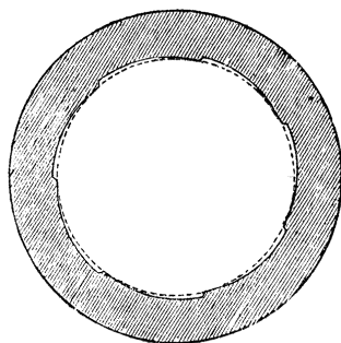
Рис. 18. Косая или однобокая нарезка.
