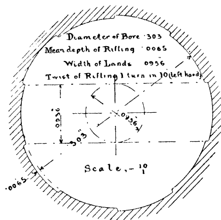
Рис. 24. Энфильдская нарезка образца 1895 г.
