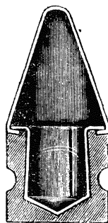
Рис. 15. Тоже для «фавнетты» более острая.
