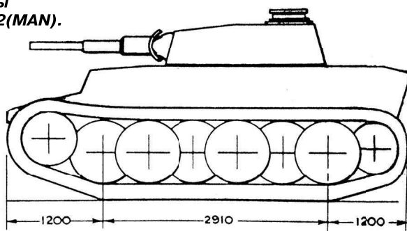
Проект фирмы Daimler-Benz — VK 2001(D).
