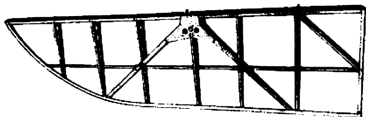
Рис. 6. Элерон (полотняная обтяжка снята)
