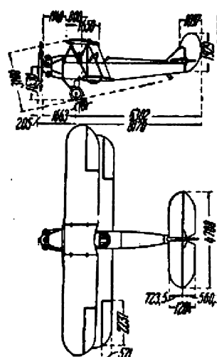
Рис. 4. Основные данные самолета У-2—М-11
