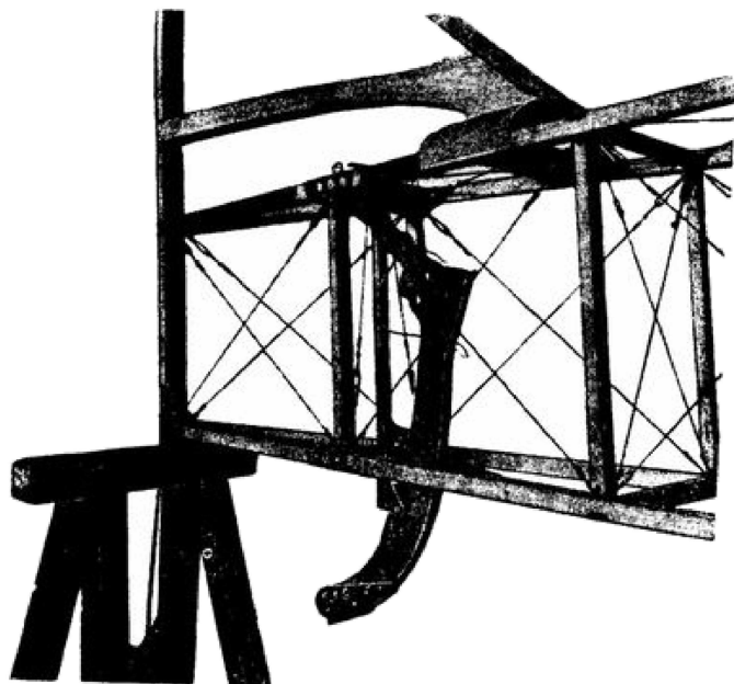
Рис. 13. Костыль
