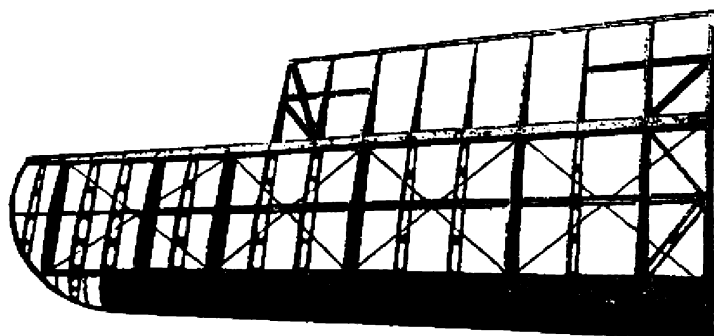
Рис. 5. Крыло (полотняная обтяжка снята)
