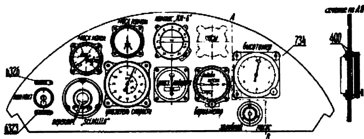
Рис. 10. Приборная доска
