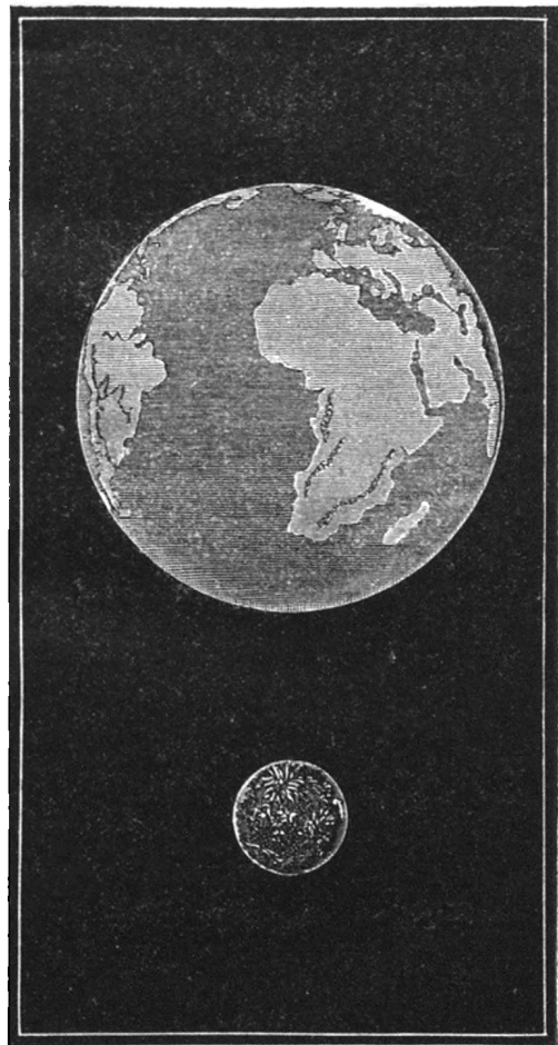
Рис. 6. Сравнительная величина Земли и Луны.
