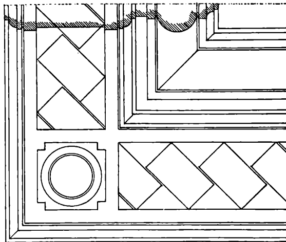
Детальный рисунокъ части той же двери и наличника.
