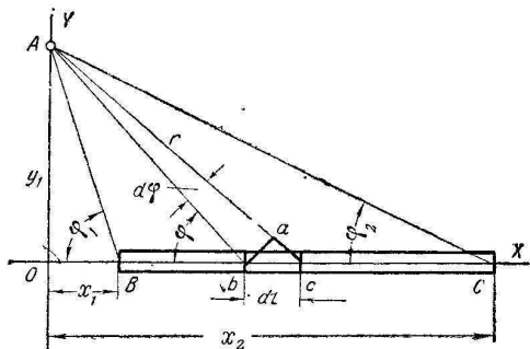
Фиг. 5. Действие вихревого отрезка.
