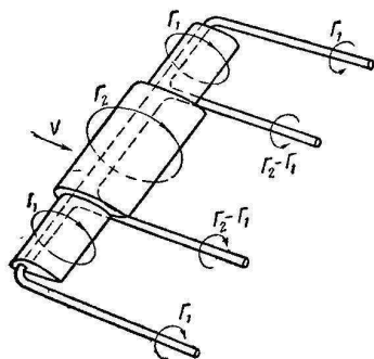
Фиг. 8. Крыло с уступами.
