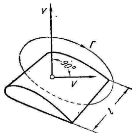
Фиг. 6. К теореме Н. Е. Жуковского.
