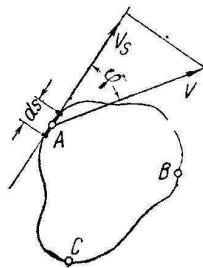
Фиг. 1. Циркуляция скорости.
