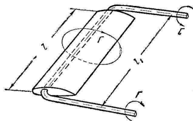
Фиг. 7. Крыло с П-образными вихрями.
