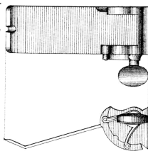
Рис. 32. Гессенскій прицѣль Литтихск. штуцера.
