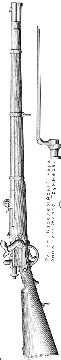
Рис. 58. Драгунская винтовка сист. Жилле-Труммера.
