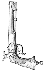
Рис. 41. Ударный офицерский пистолет.
