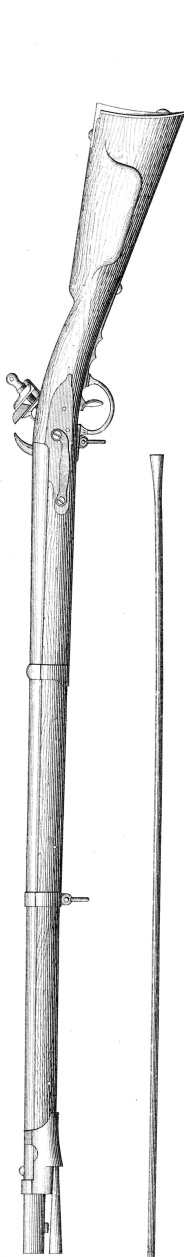
Рис. 17. Кремневое драгунское и кирасирское ружье обр. 1828 г.
