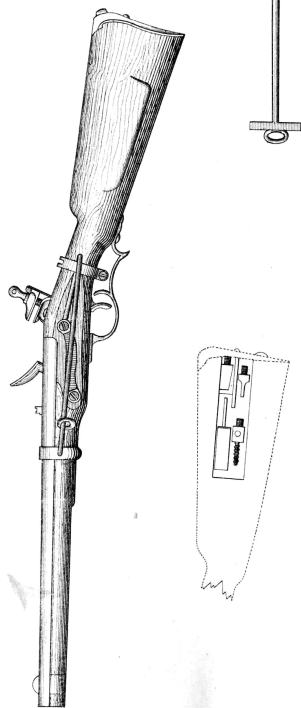
Рис. 22. Кремневый Кавалерійскій штуцеръ обр. 1839 г.
