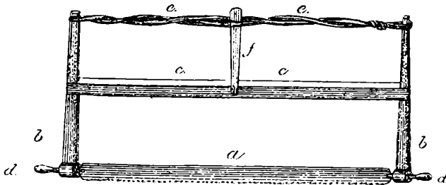
Рис. 14. Обыкновенная лучковая пила.
