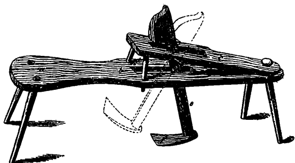
Рис. 10. Станокъ для работы стругомъ.
