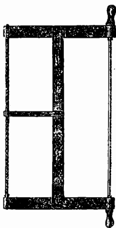
Рис. 18. Поворотная пила.
