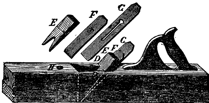
Рис. 7. Фуганокъ.
