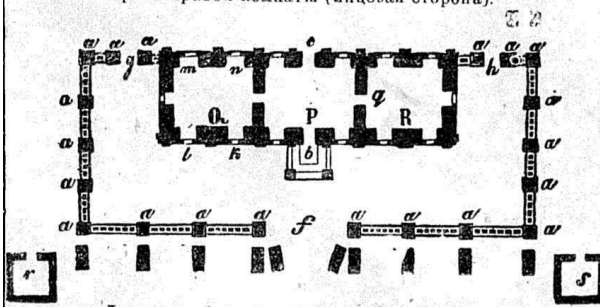
и. планъ Ледяного дома: a, a, a —ледяная рѣшетка; b —крыльцо; P —спяни; R —правая комната; Q —лѣвая комната; f —главный вѣрота; g, h —заднія вѣрота; m, n, k, l —окна; c —задняя дверь; r, s —пирамиды.
