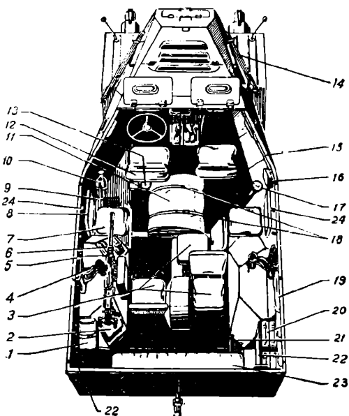
Рис. 4. Отделение управления и боевое отделение:
