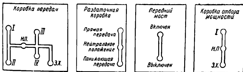
Рис. 7. Схема положений рычагов коробки передач, раздаточной коробки и коробки отбора мощности
