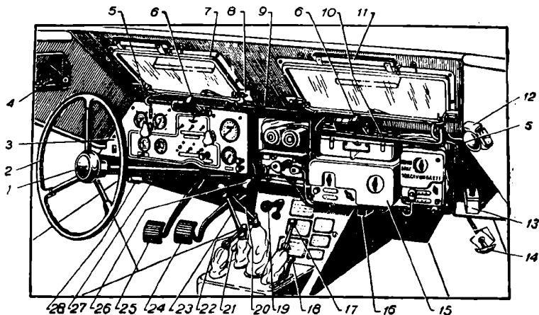
Рис. 5. Органы управления и приборы:
