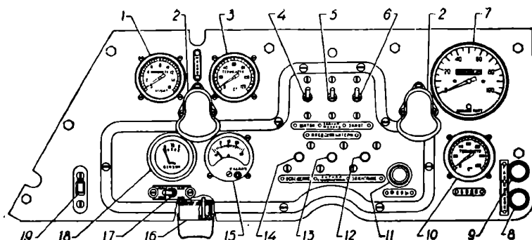
Рис. 6. Щиток приборов:
