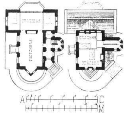
Планы.
