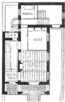
КОТТЭДЖЪ въ ST.-ANDRAU. Арх. WILLIAM.
