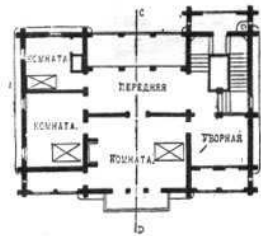
Планъ 2-го этажа.
