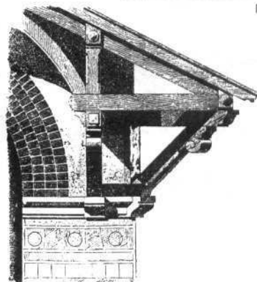
Деталь фронтона.
