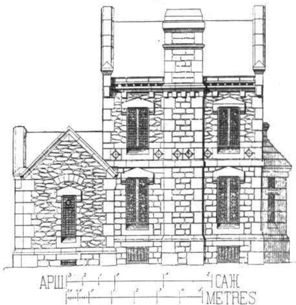
Западный фасадъ.
