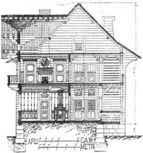
Разрѣзъ.
