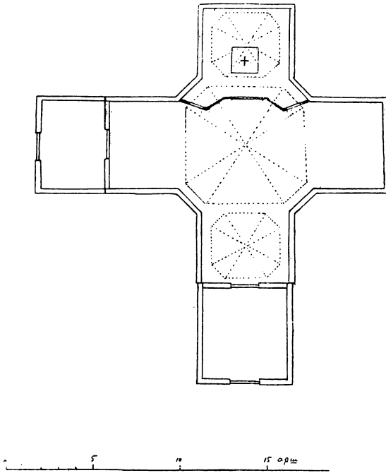
Планъ старой церкви с. Паланки Ямпольскаго уѣзда.
