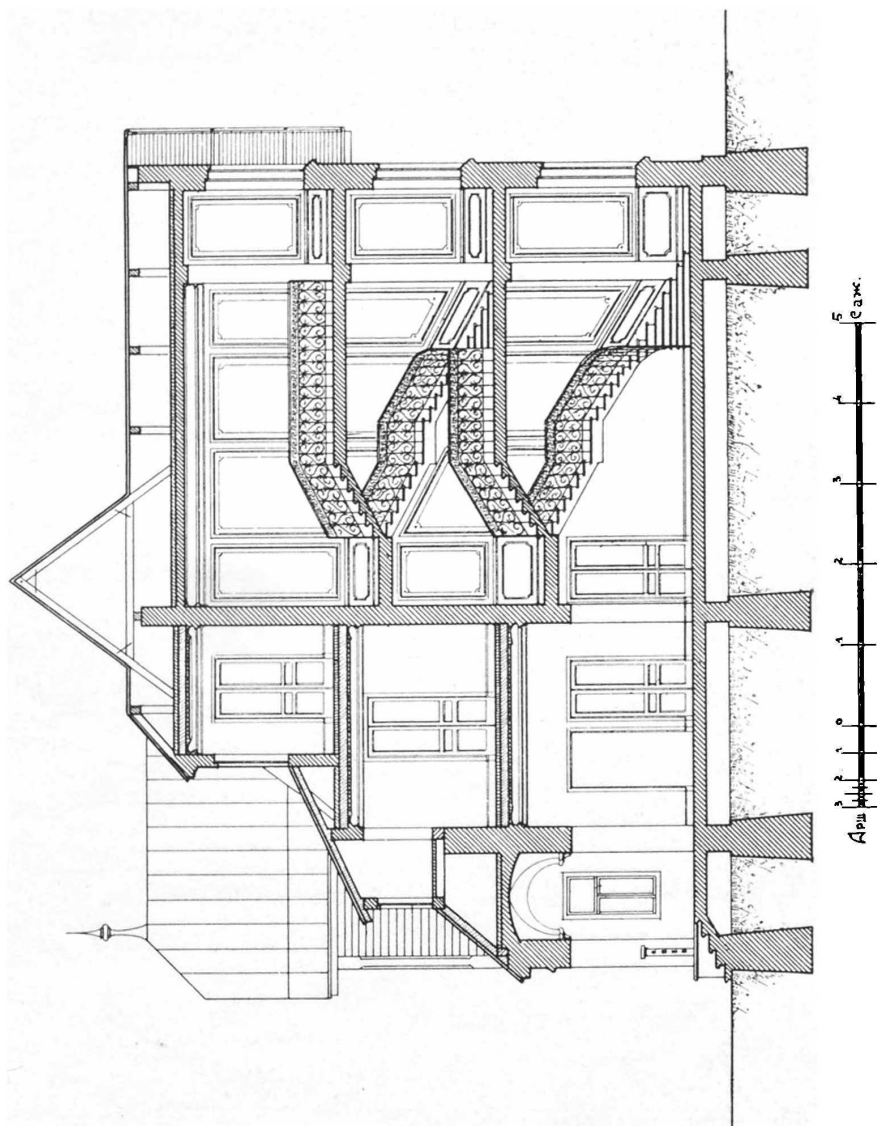
Проектъ 1. Загородный домъ. Разрѣзь по А—В.
