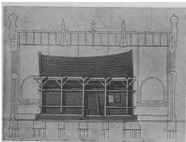
Разрѣзъ каменнаго строенія и домина Петра I. Въ современномъ видѣ.
