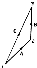
Рис. 1. Сложение двух векторов.
