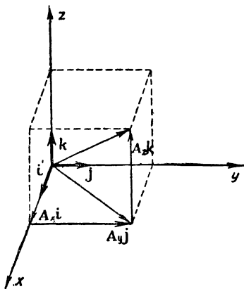
Рис. 6. Ортогональные единичные векторы i, j, k .
