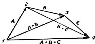
Рис. 3. Сложение трех векторов.
