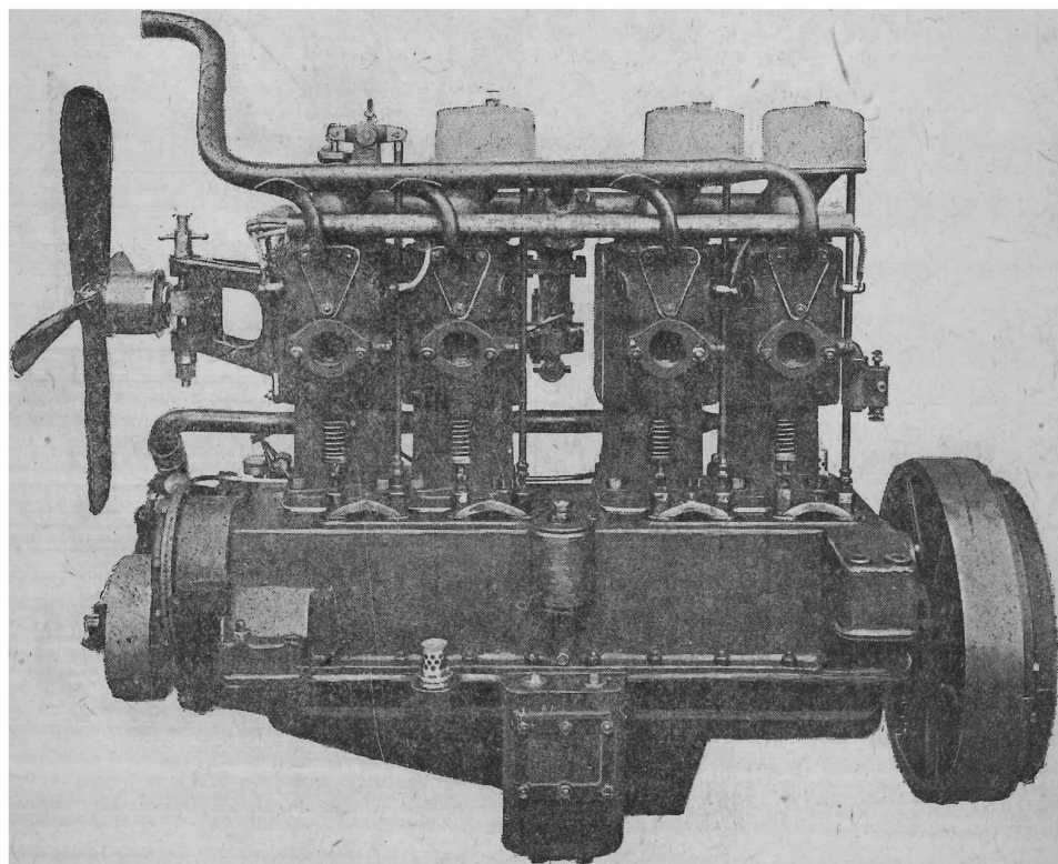
Фиг. 6. Двигатель (вид слева, по ходу)
