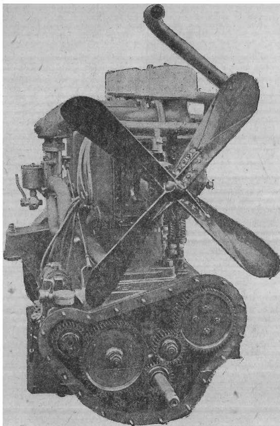
Фиг. 5. Двигатель. Передняя крышка картера снята. Видны шестерни распределения
