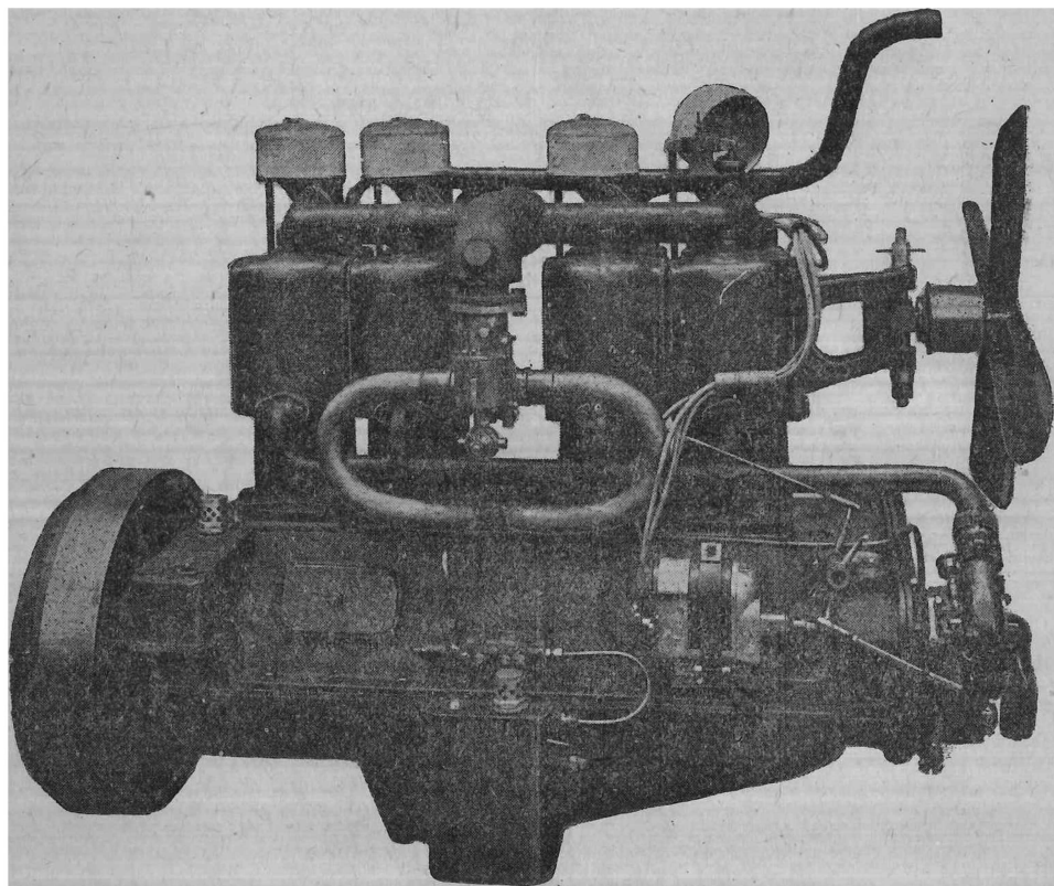
Фиг 7. Двигатель (вид справа, по ходу)
