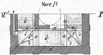
План западной части свода.
