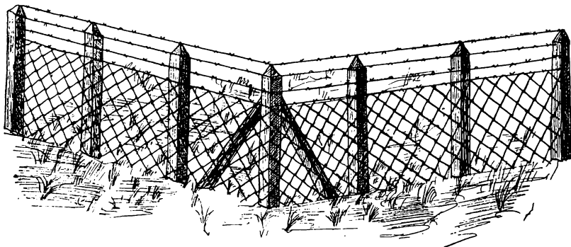
Рис. 2. Общій видъ готовой сѣтчатой изгороди.
