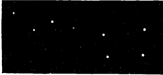
Семь самыхъ большихъ звѣздъ созвѣдія Большой Медвѣдицы.
