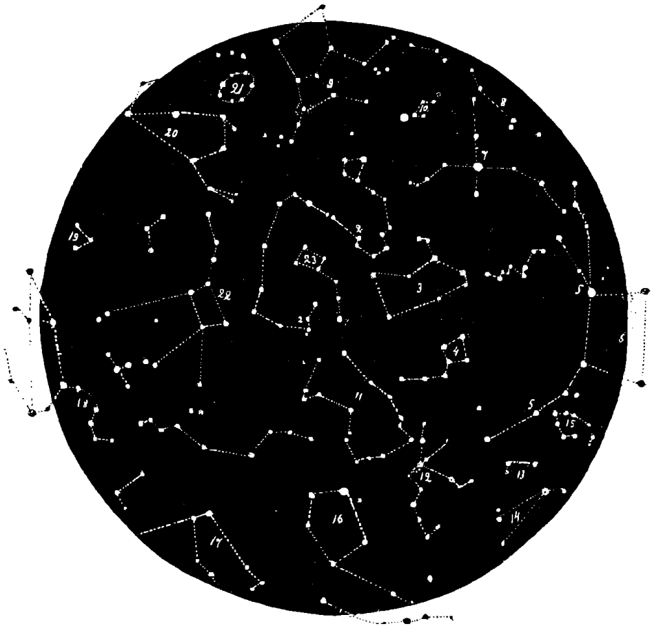
Главнѣйшія созвѣздія сѣвернаго полушарія неба.
