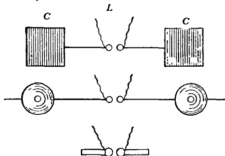
Фиг. 3. Различные виды вибратора Герца
