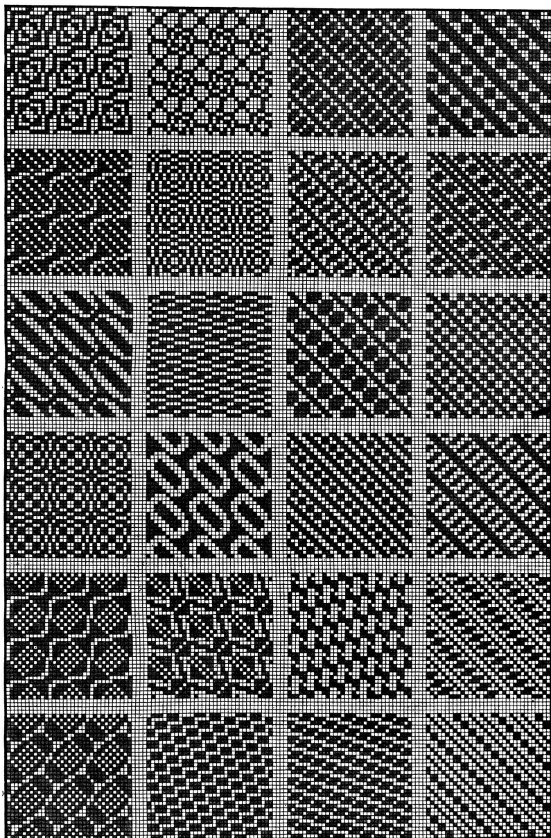
Одиннадцатиремизныя переплетенія.
