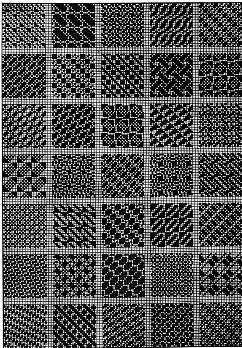
Девятиремизныя переплетенія.
