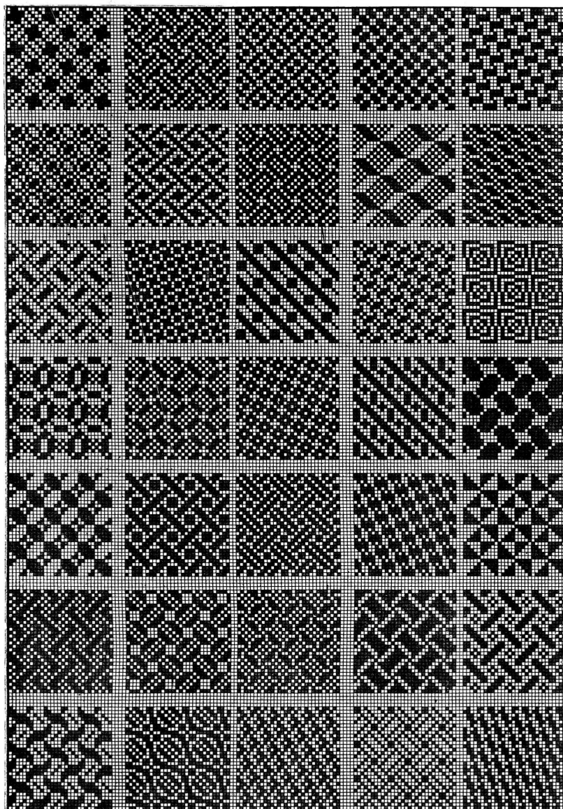
Десятиремизныя переплетенія.
