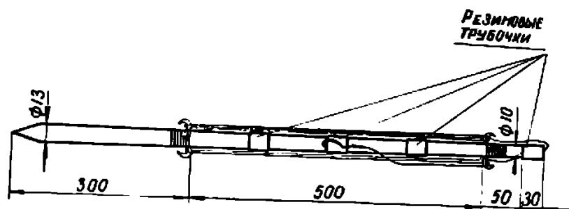
Рис. 1. Удильник для донной удочки
