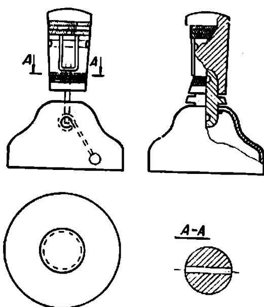
Рис. 3. Оснащение колокольчика деревянной колодочкой с проволочкой для подвешивания на леску
