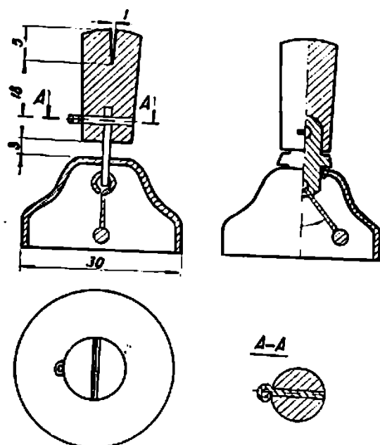
Рис. 4. Способ подвешивания колокольчика с деревянной колодочкой взажим
