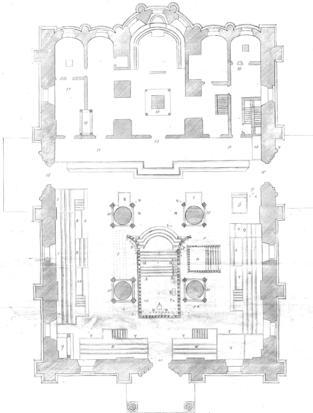
Описание и план здания Успенскаго Собора въ Новгородѣ 1730 трипротрашеви ея Императорскаго Величества.
