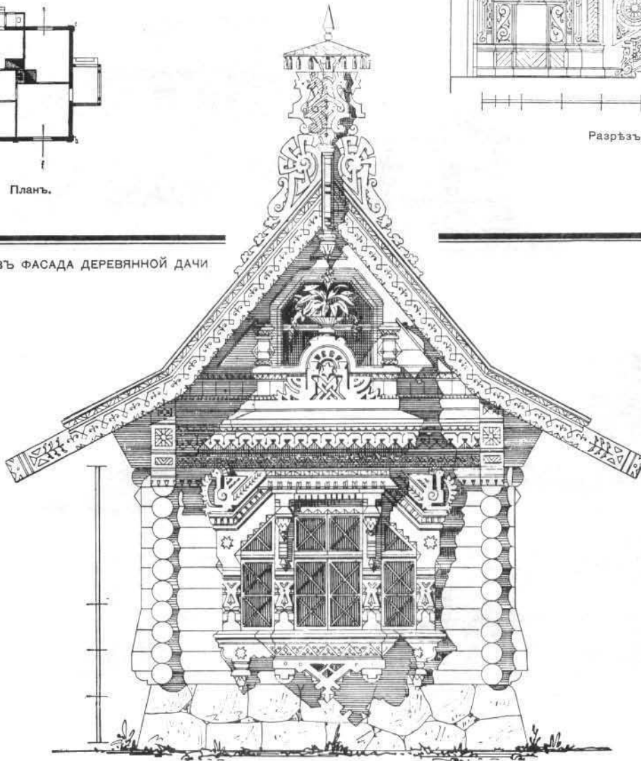
Задній фасадъ.
