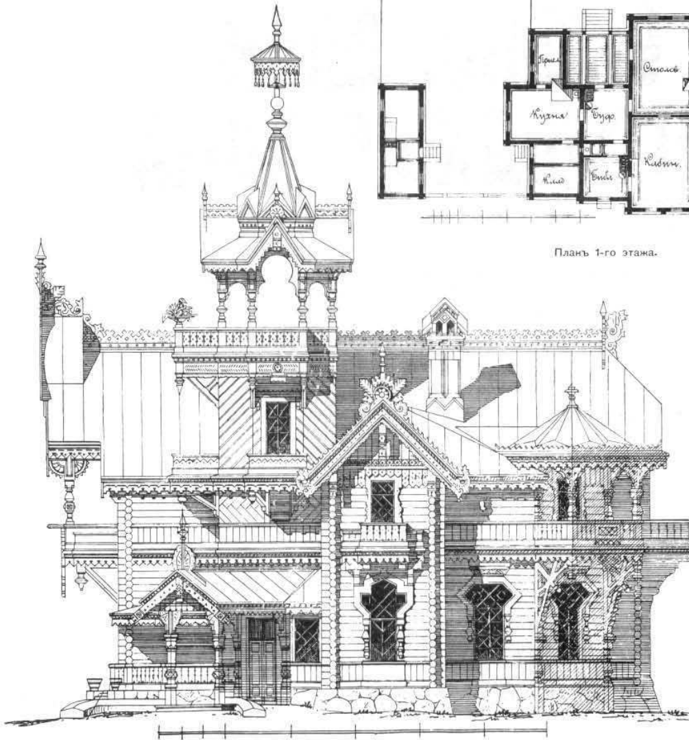
Боковой фасадъ.
