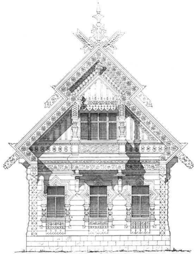
Деталь фасада.
