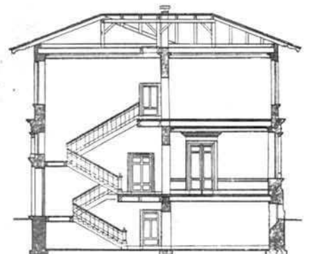
Разрѣзъ.
