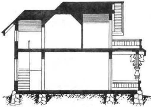
Разрѣзъ.
