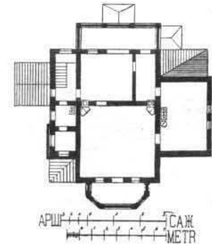
Планъ 2-го этажа.
