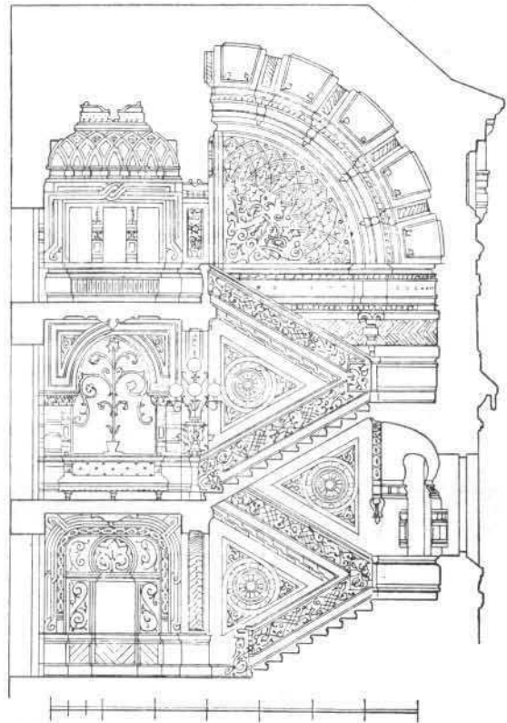
Разрѣзъ.
