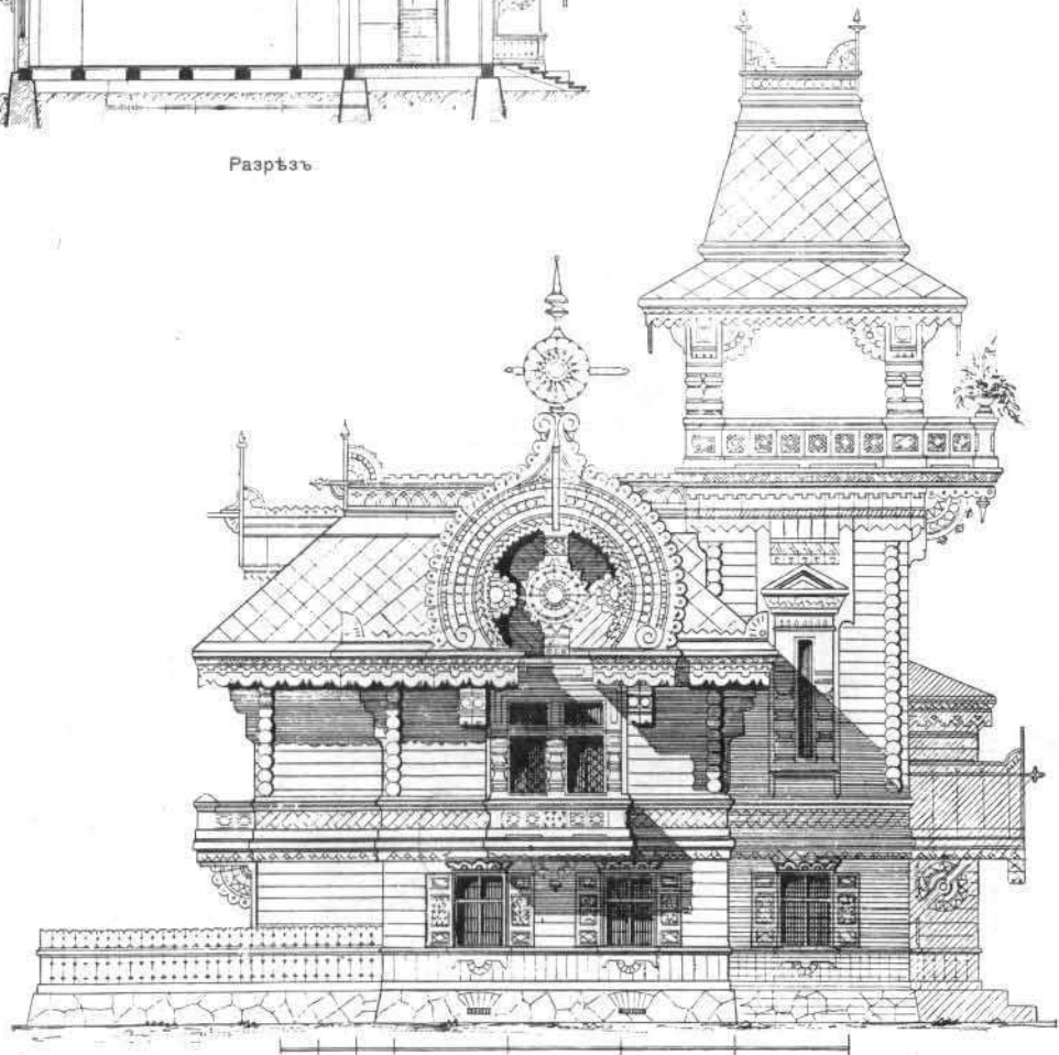
Фасадъ.
