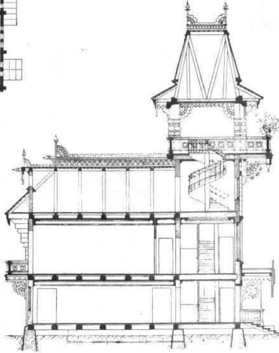
Разрѣзъ.
