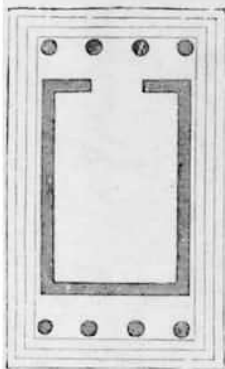
Рис. 4 (§§ 8, 15). Амфипростиль.
