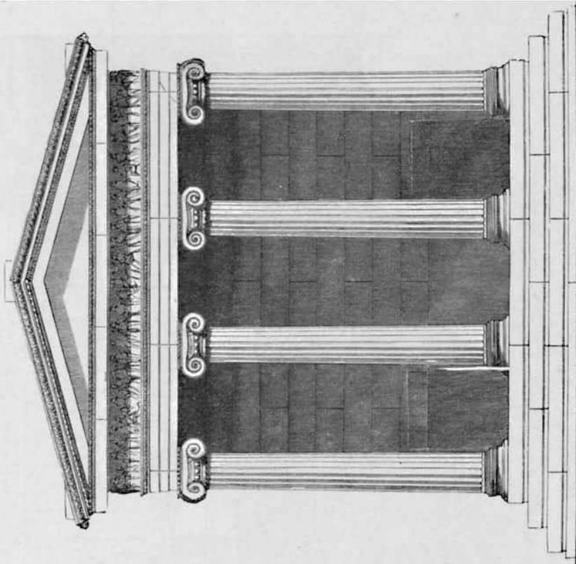
Рис. 5 (§§ 8, 12, 15). Храм Афина-Нинге передо. Акрополь ил. Афин.
