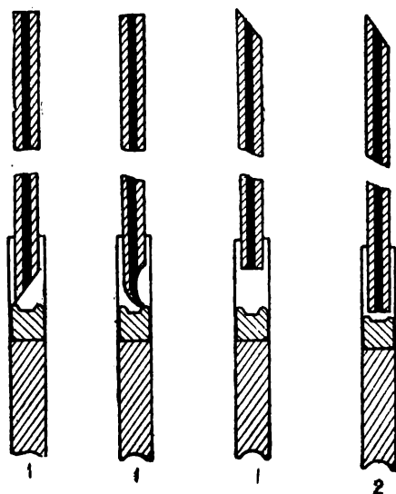
Рис. 5. Ввод шнура в капсюль:
