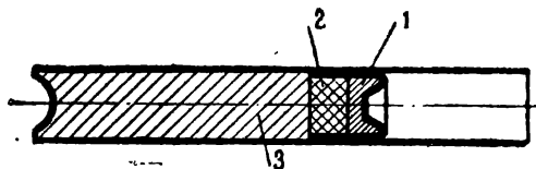
Рис. 2. Капсюль-детонатор ТАТ № 8:
