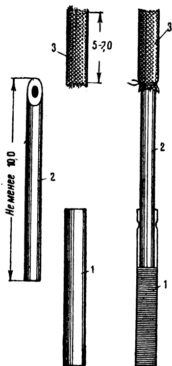
Рис. 4. Зажигательная трубка:
