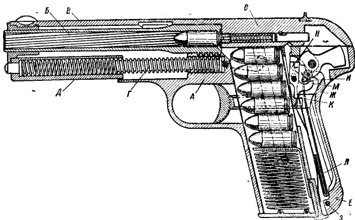
Рис. 4. Пистолет Браунинга калибром 9 мм.
