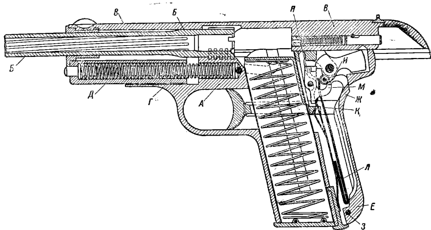
Рис. 5. Пистолет Браунинга калибром 9 мм.
