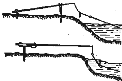
Рис. 2. Полудонка для ловли на течении
