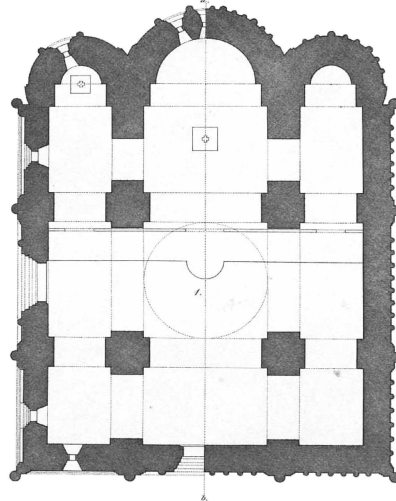
ФАСАДЫ И ПЛАНЪ ДМИТРІЕВСКАГО СОВОРА Въ Свѣтлѣ на Тѣмнѣ.
