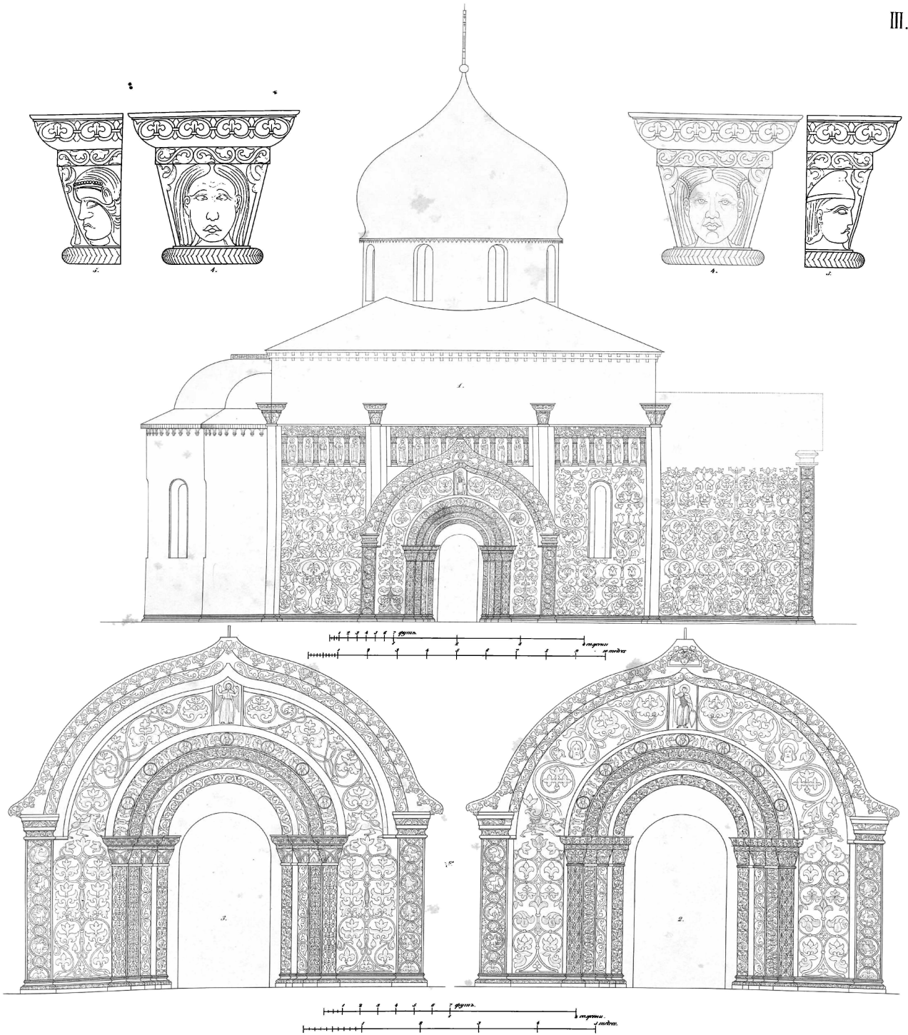
ПОРТИКИ и ВОКОВОЙ ФАСАДЪ ЦЕРКВИ С В ГЕОРГІЯ в Кремлѣ Москвитинъ.
