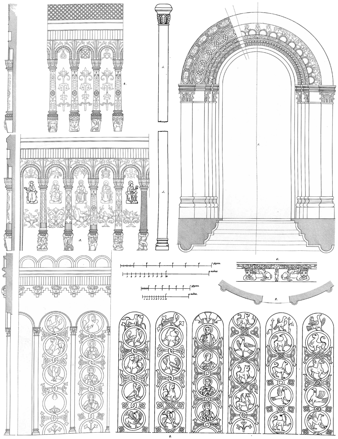
ДЕТАЛИ ДМИТРИЕВСКАГО СОВОРА, ВО ВЛАДИМИРЬ.
