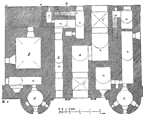
Планъ I-го этажа.
