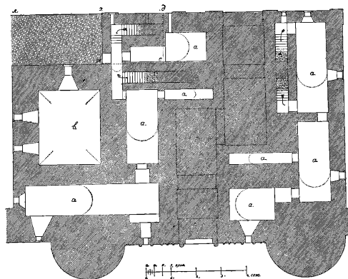
Планъ II-го этажа: (антресоль).
