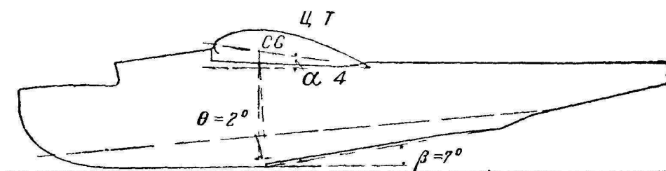
Фиг. 3. Положение центра тяжести относительно редана.
