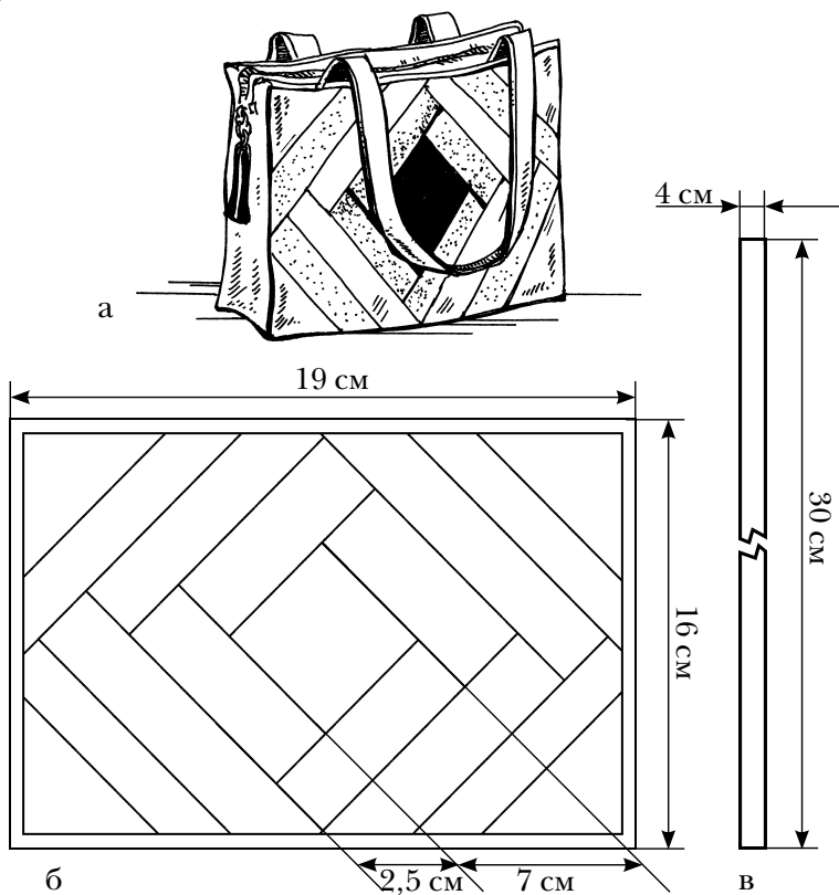
Рисунок 1. Болоньевая сумка: а) готовое изделие; б) схема 1; в) схема 2
