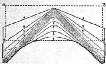
Фиг. 6. Послѣдовательное измѣненіе формы желѣзной (и стальной) полосы при полученіи углового желѣза.
