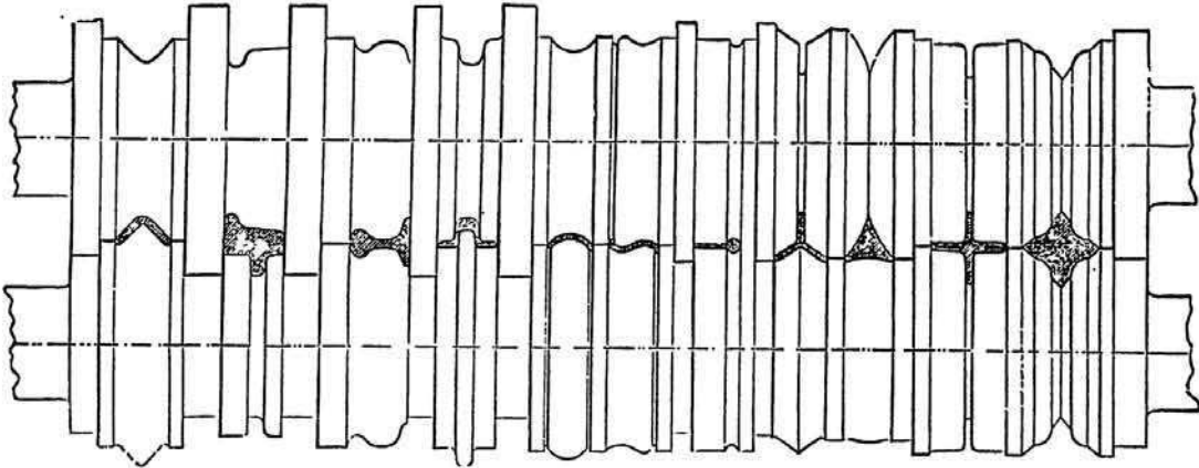
Фиг. 3. Отдѣльные ручки прокатныхъ вальцовъ для полученія различныхъ сортовъ фасоннаго желѣза (и стали).
