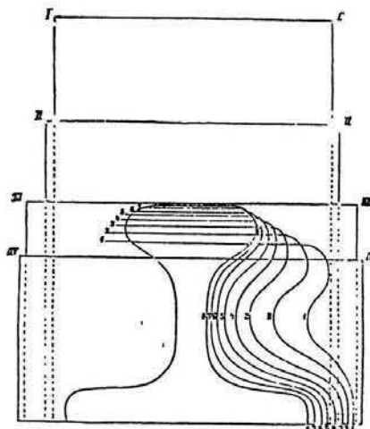
Фиг. 5. Послѣдовательное измѣненіе сѣченія пакета при прокаткѣ рельсового желѣза (и стали).
