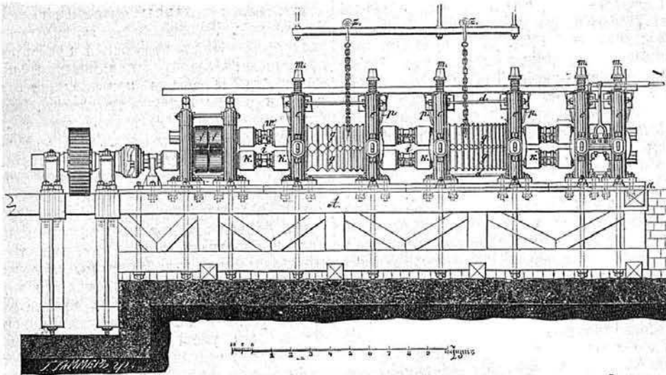
Фиг. 1. Прокатный станъ для полученія сортового желѣза (и стали). Общій продольный видъ.
