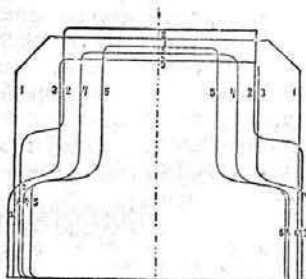
Фиг. 7. Послѣдовательное измѣненіе формы желѣза (и стали) при прокатываніи таврового желѣза.
