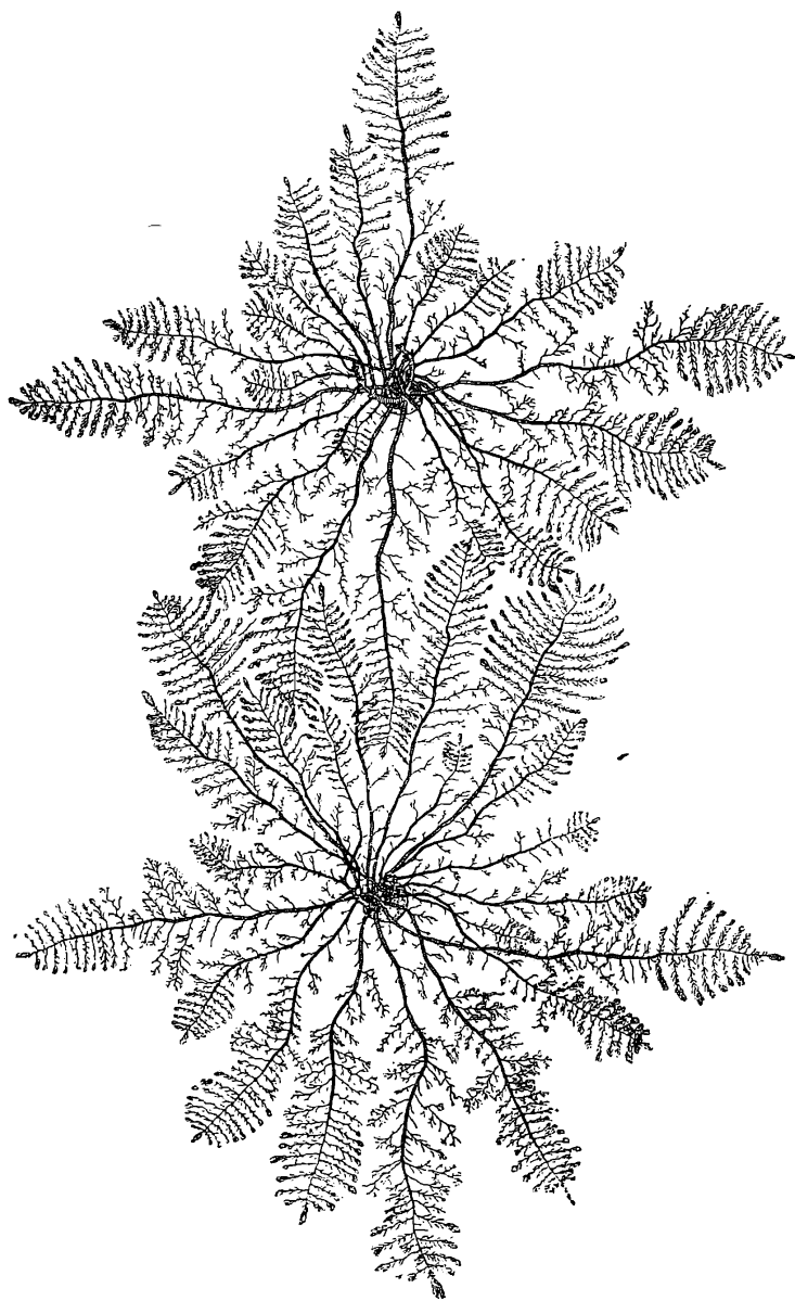
Рис. 2. Видъ сверху вполне развитыхъ верховыхъ корней.
